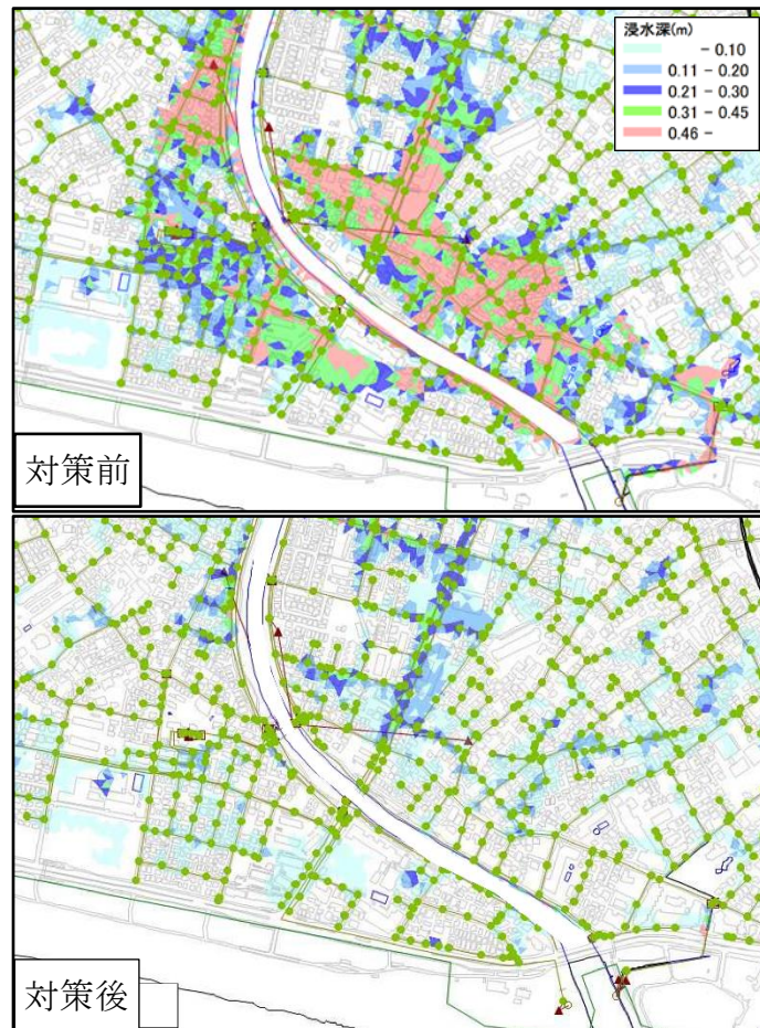
図33 浸水シミュレーション対策前後比較（10年確率降雨 \times 1.1 ）
