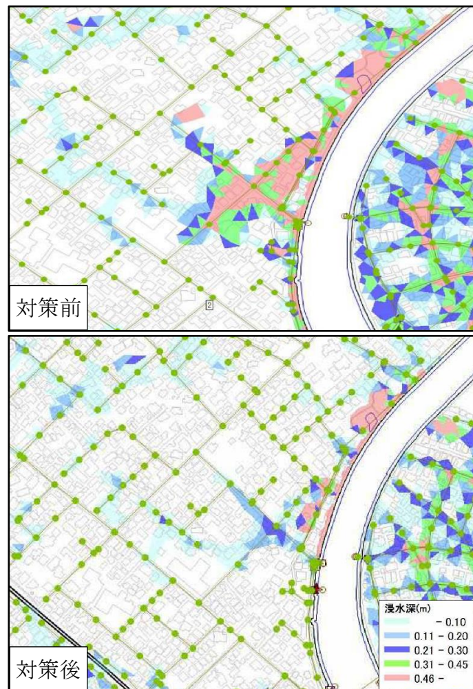
図28 浸水シミュレーション対策前後比較（10年確率降雨×1.1）
