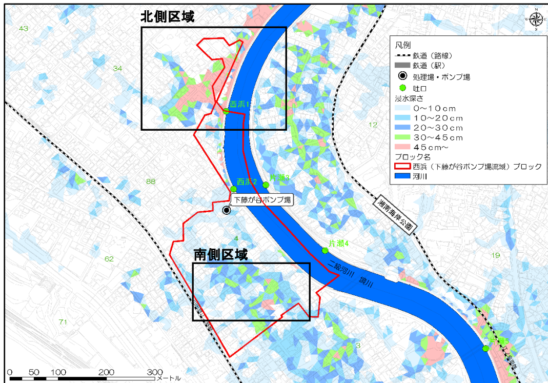
図27 西浜（下藤が谷ポンプ場流域）ブロック全体図（10年確率×1.1）
